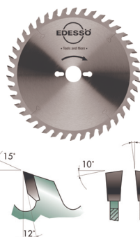
Zuschneidesägeblatt Hartmetall lame de scie à débiter métal dur
