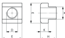
T-Nutensteine, ohne Schrauben tasseau à T sans vis
