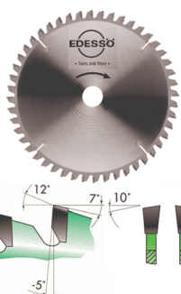
Profi-Kreissägeblatt Hartmetall lame de scie circulaire pro métal dur
